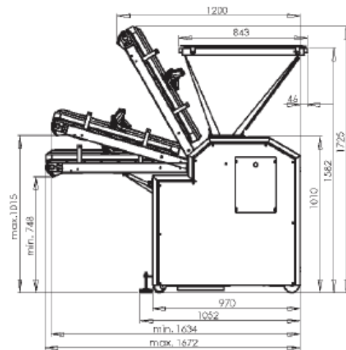
CPL MAXI 2 P
