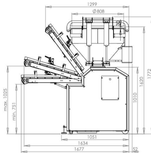
CPL MAXI 4 P
