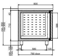
SEZ. A-A
