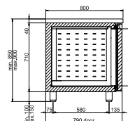
SEZ. A-A
